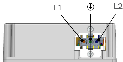
“-9P” Input
