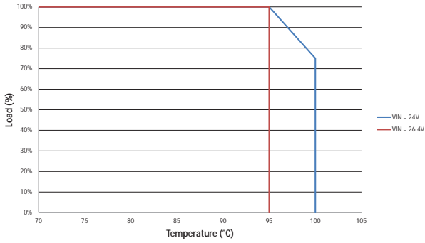
MGJ1D241505MPC
