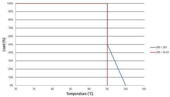
MGJ1D241905MPC
