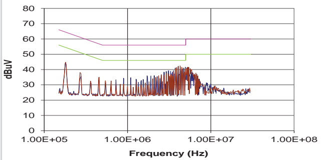
MGJ1D121905MPC
